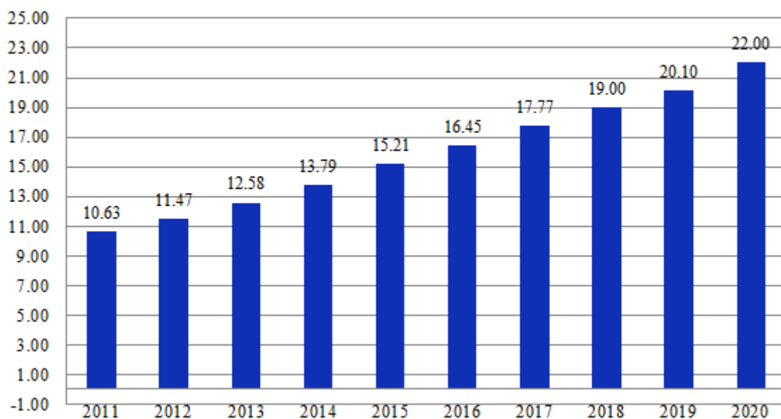
近十年我国发电装机总容量（单位：亿千瓦时）
